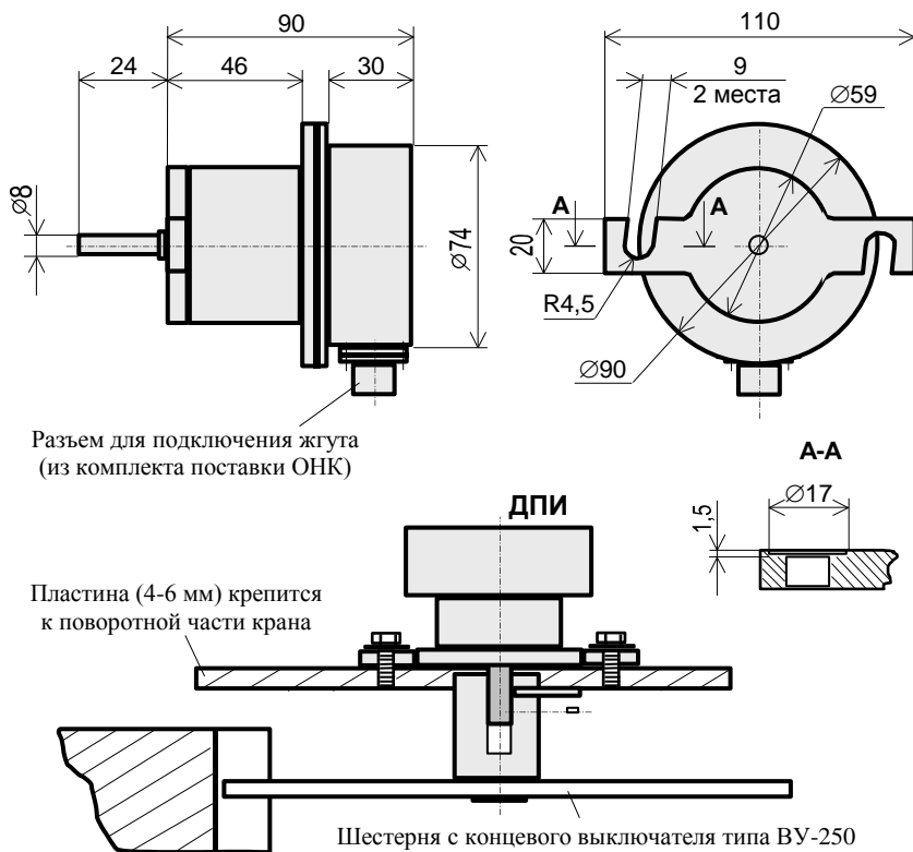
Рисунок 17 - Установка ДПИ
