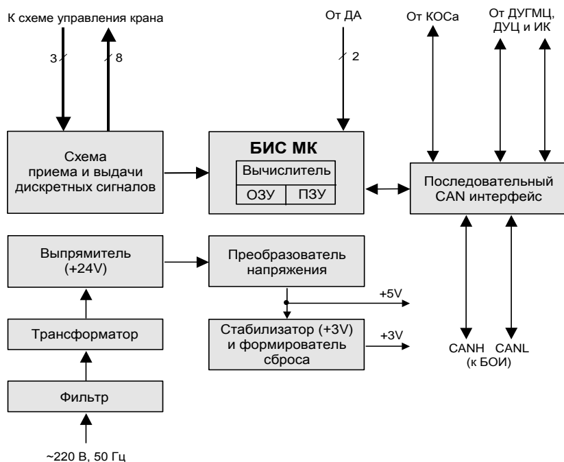
Рисунок 4 - Блок-схема БПК
